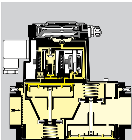
CG 25-30
